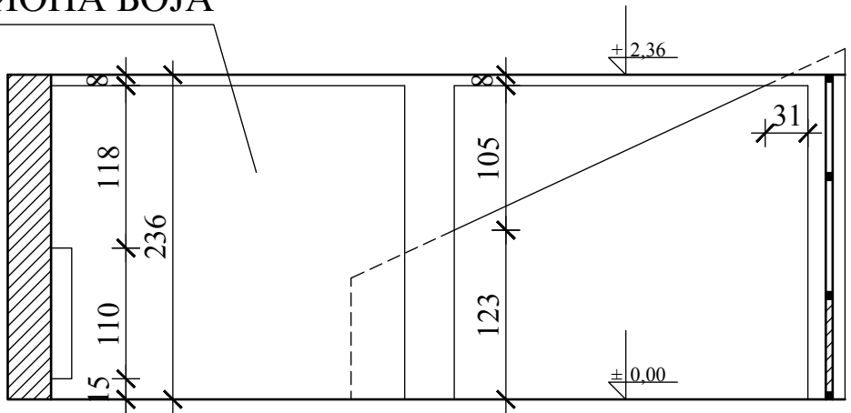
ПРЕСЕК Б-Б
