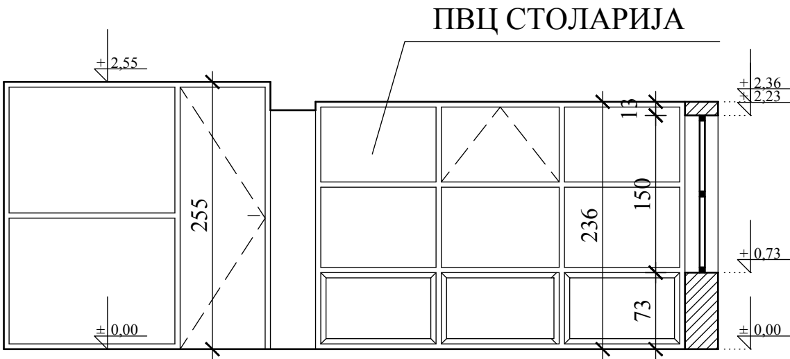
ПРЕСЕК В-В
